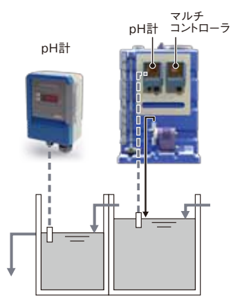
排水フロー
