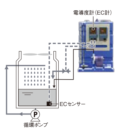
クーリングタワーフロー
