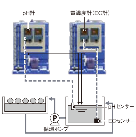
養液フロー
